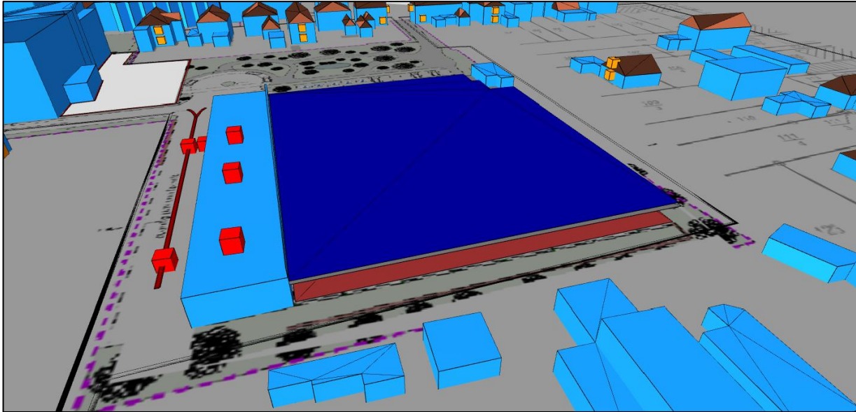
Abbildung 5: 3D-Ansicht aus dem Schallausbreitungsmodell.
